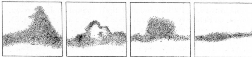
FIG. 1.—1840. Beer and Mædler. FIG. 2.—1856. W. de la Rue. FIG. 3.—1858. Secchi. FIG. 4.—1875. Holden.
